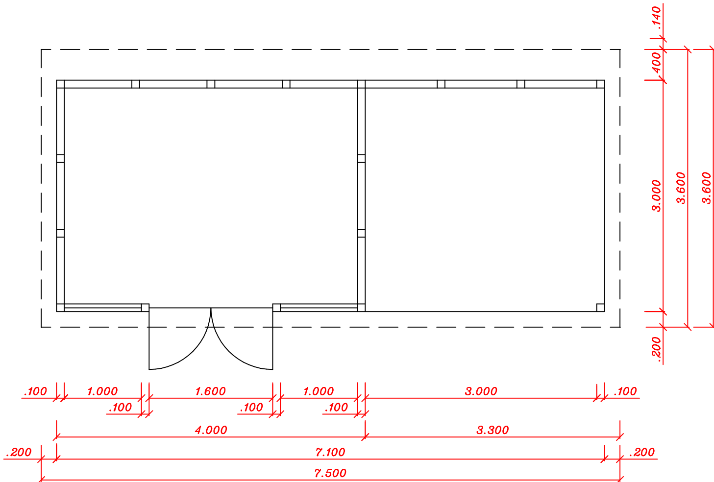
Grundriss
