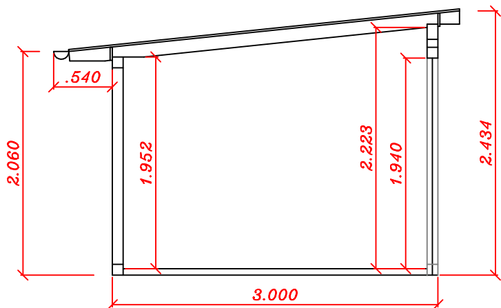
Schnitt
