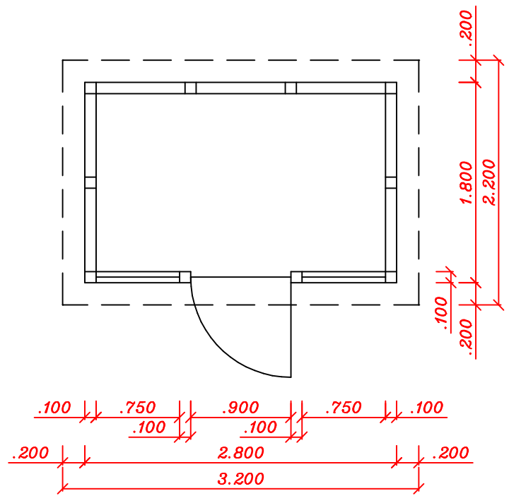
Grundriss
