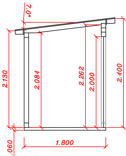
Schnitt
