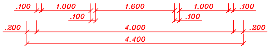
Grundriss
